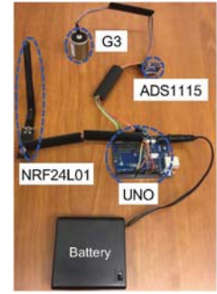
Fig. 6. Controller B.
