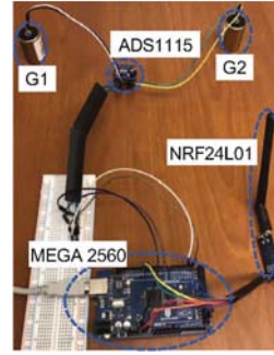
Fig. 5. Controller A.
